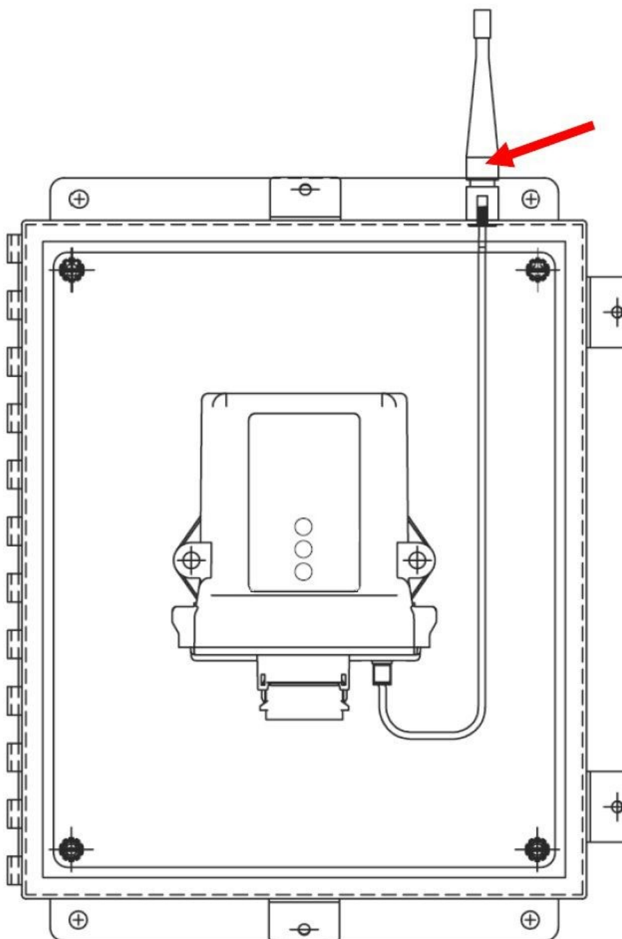
Obr. 1: Montáž přijímače CAN-2 v rozvaděči a umístění vnější antény
