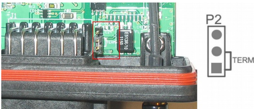
Obr. 3: Umístění propojky P2 pro zapojení zakončovacího rezistoru v přijímači
