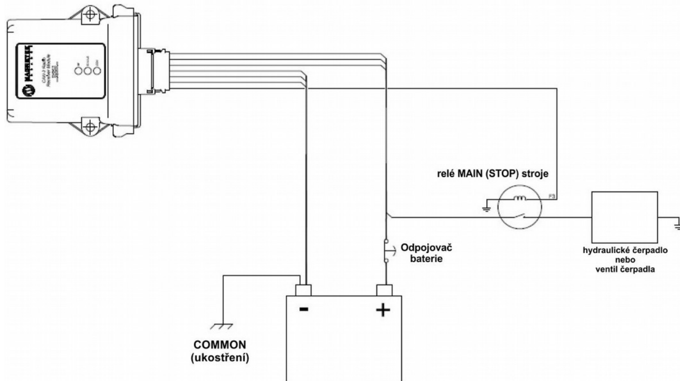
Obr. 4: Doporučené zapojení přijímače CAN-2
