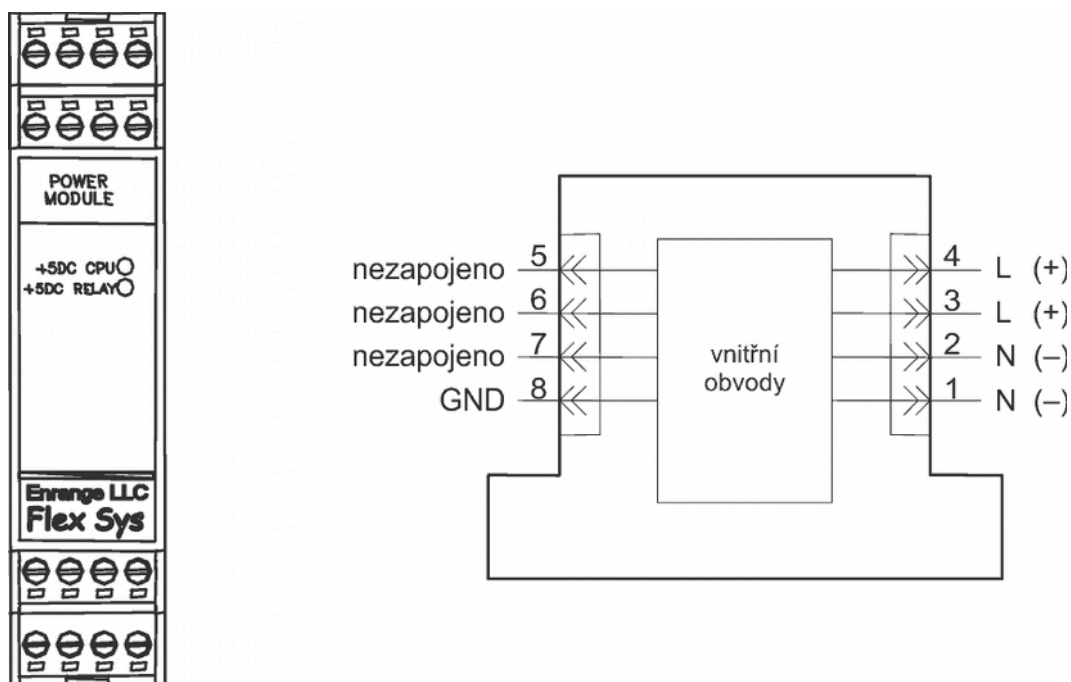
Obr. 5: Zapojení napájecího modulu
