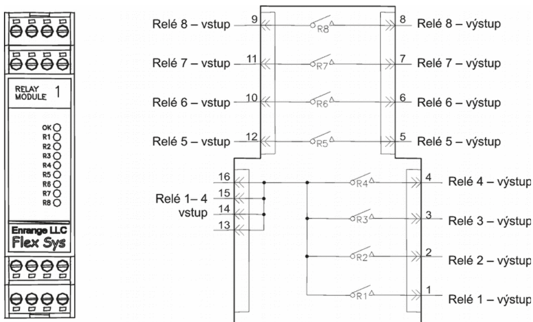
Obr. 6: Zapojení reléového modulu
